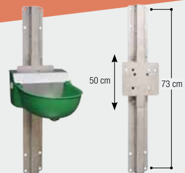
101.0433 Höhenverstellung mit Modell 130P
